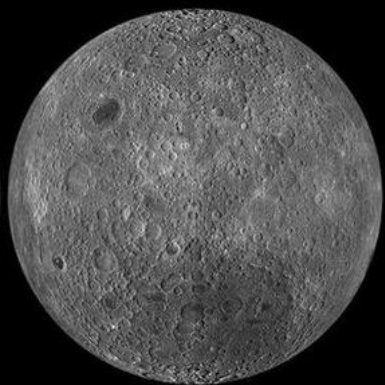
月球背面
