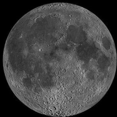
月球正面
